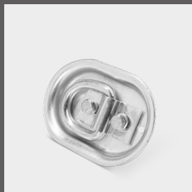
In houten vloer verzonken, gemonteerde ringen, trekkracht elk 0,2 t (4 stuks)
