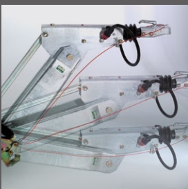
In hoogte verstelbare trekdijsel (kogelkoppeling en DIN-sjorrog niet meegeleverd)
